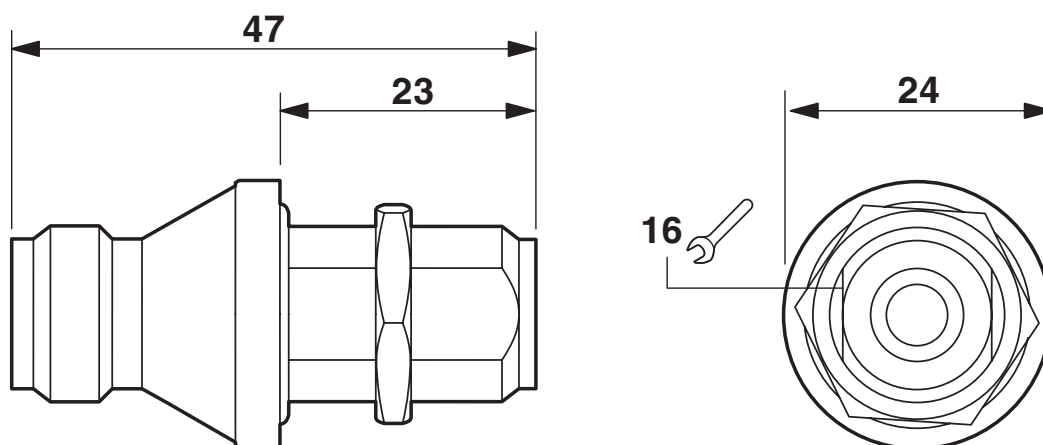
Dessin coté
