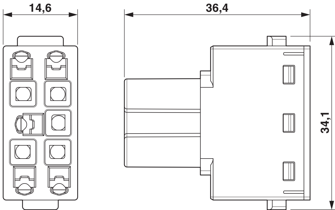
Maßzeichnung
