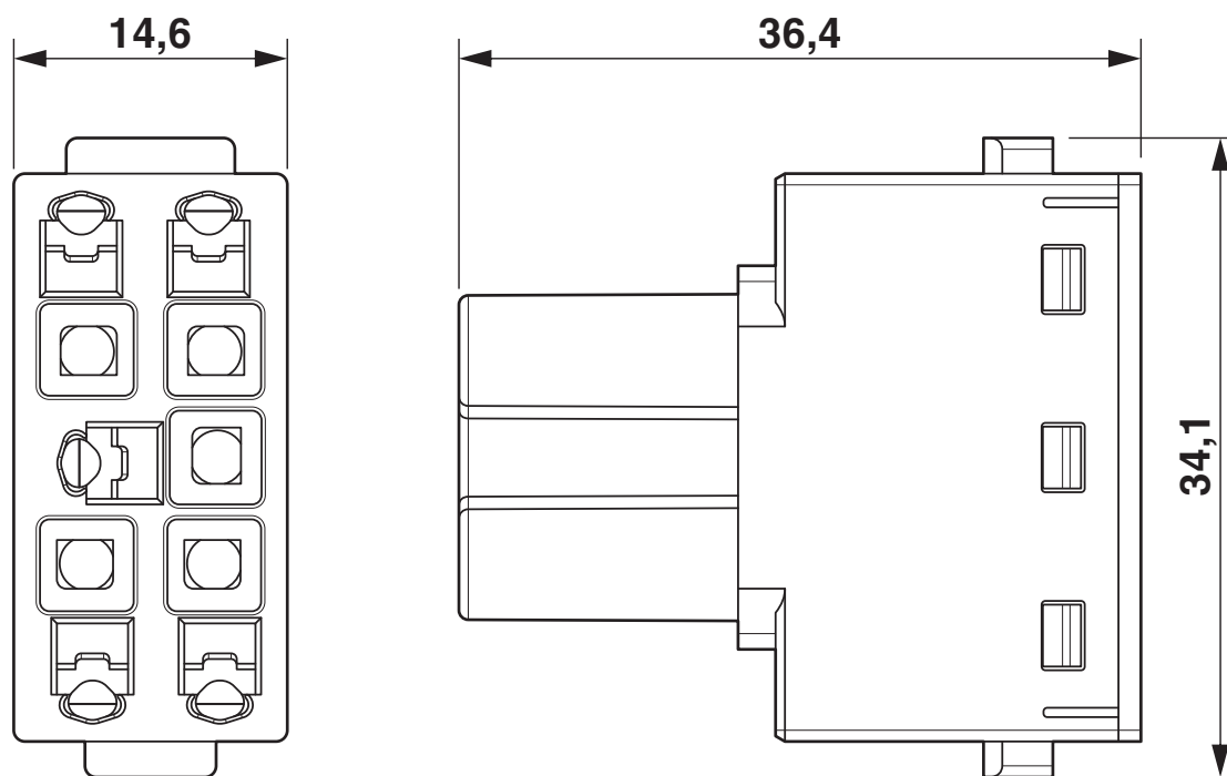
Dessin coté
