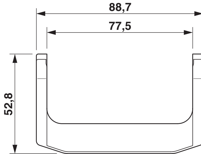
Maßzeichnung
