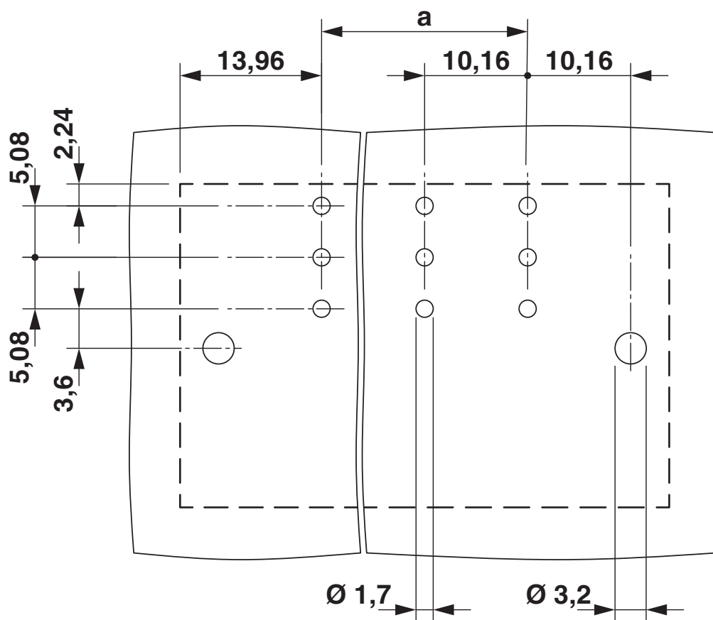
Gabarit perçage / géom. pastille soudage
