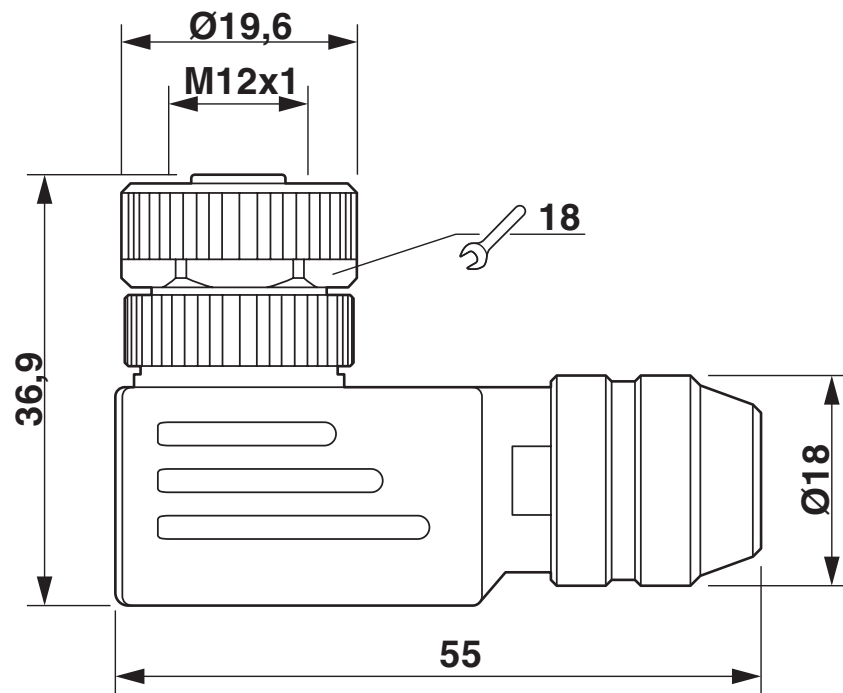
Dessin coté
