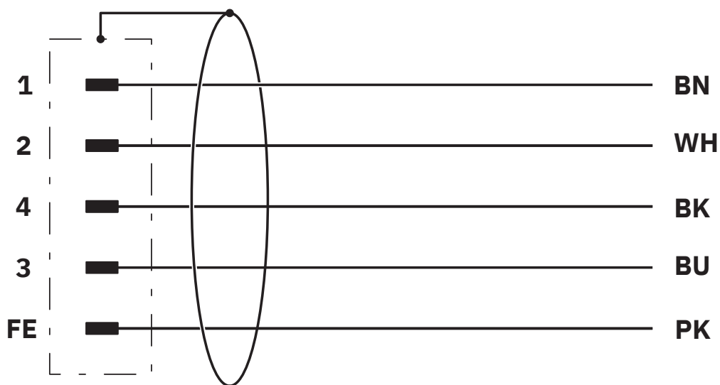
Diagrama eléctrico
