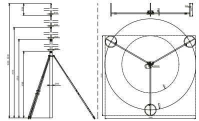
Maßbild FS T D50 1.6 6.5M AL DBS RA1435
