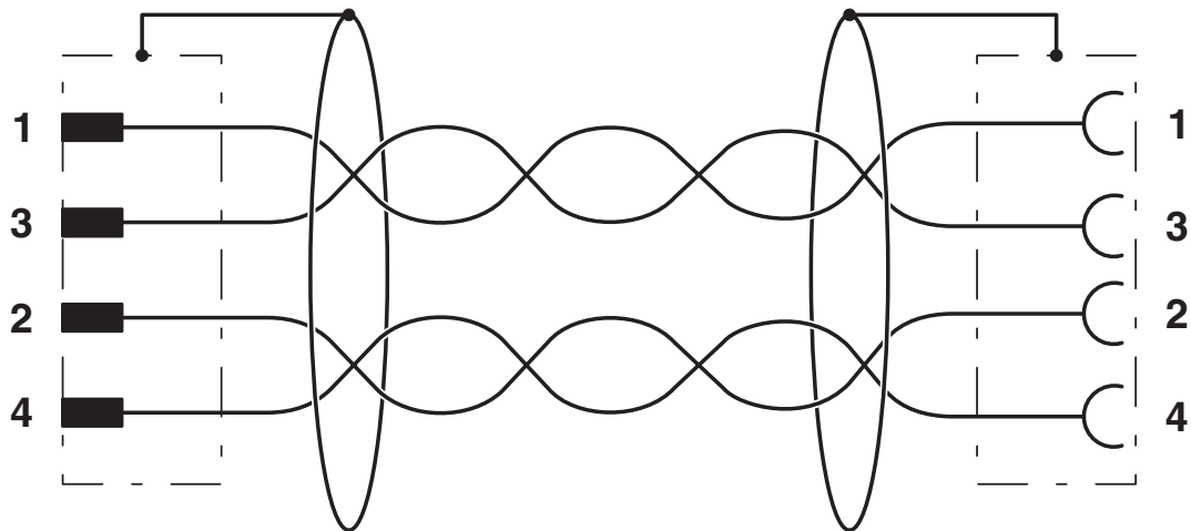
Diagrama eléctrico
