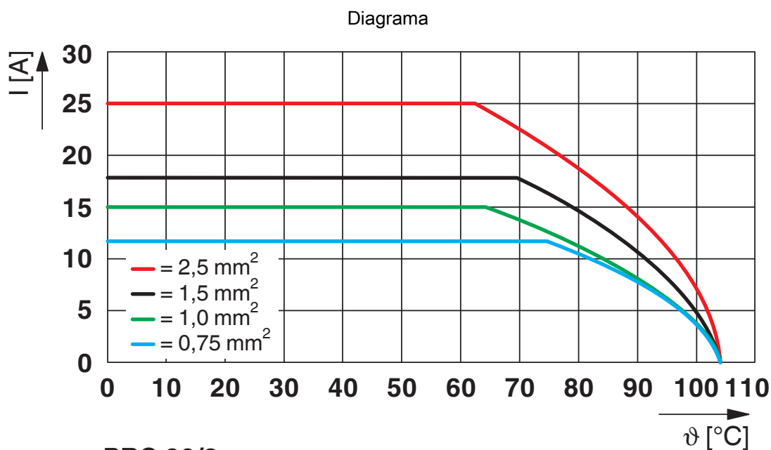
PRC 20/3... IEC 60512-5-2 / 2 conductors
