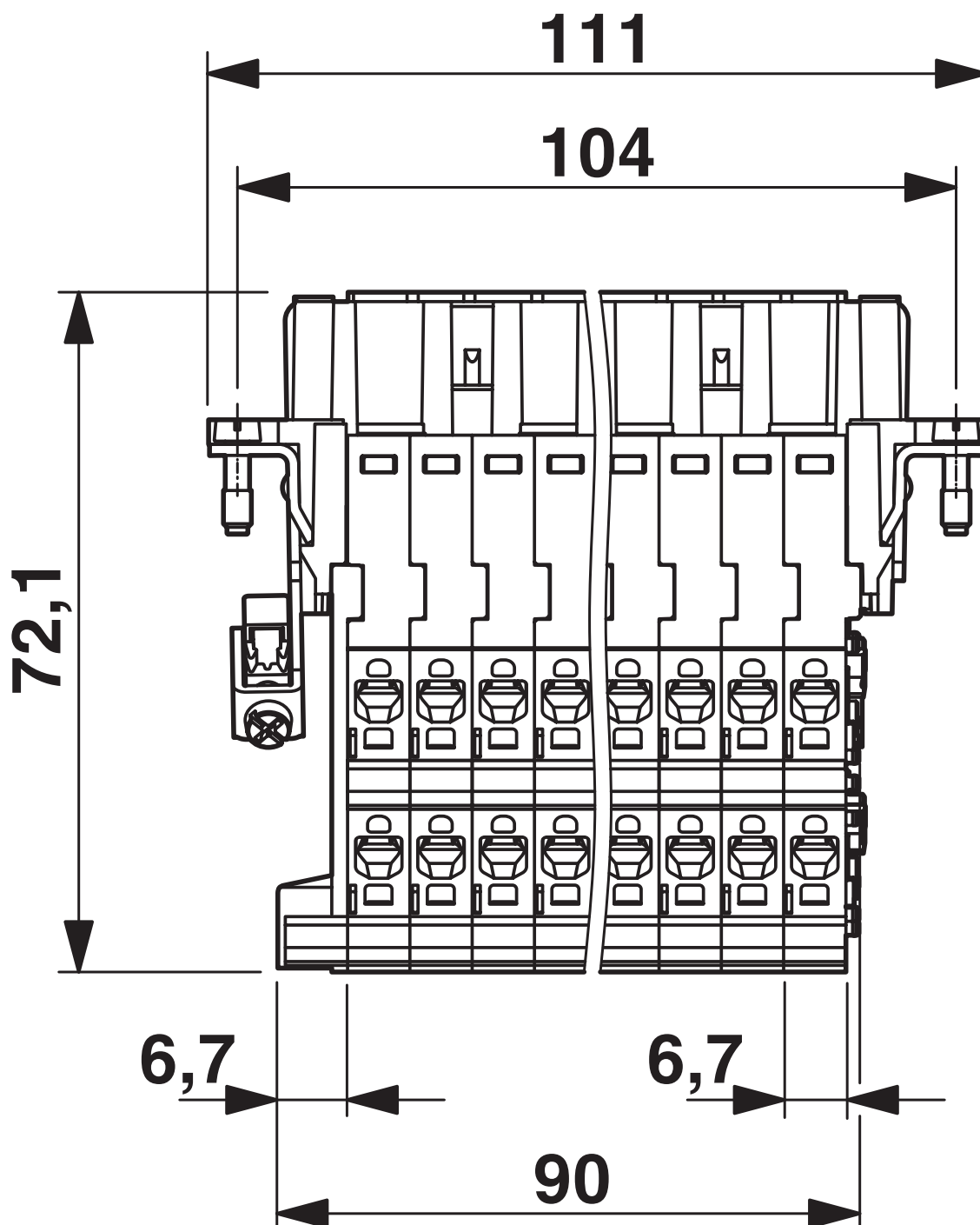
Dessin coté
