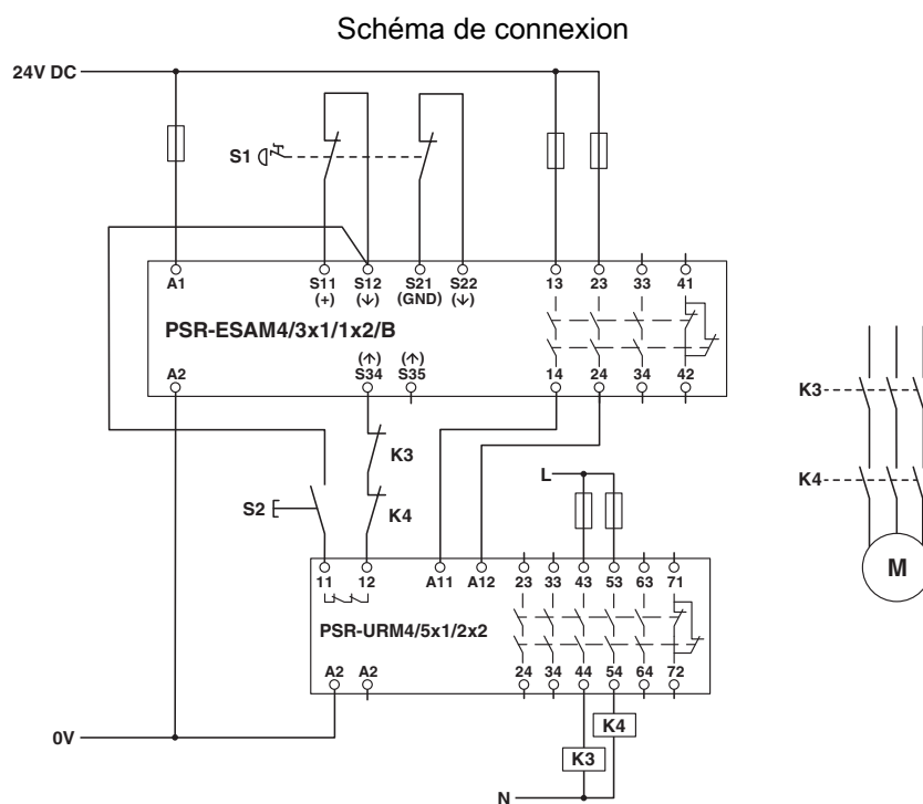
Raccordement à deux canaux avec intégration du circuit report de signalisation et contacts à surveillance externe
