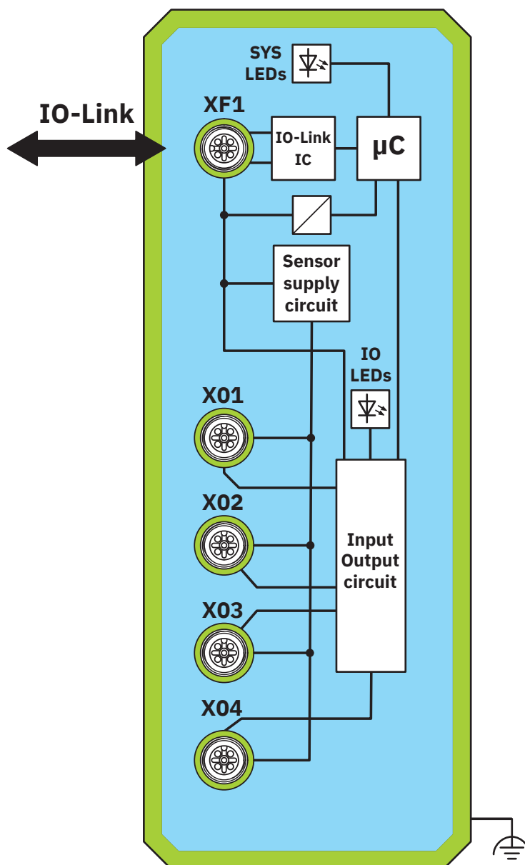
Schéma fonctionnel
