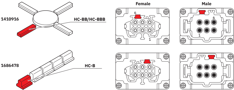
Plano esquemático
