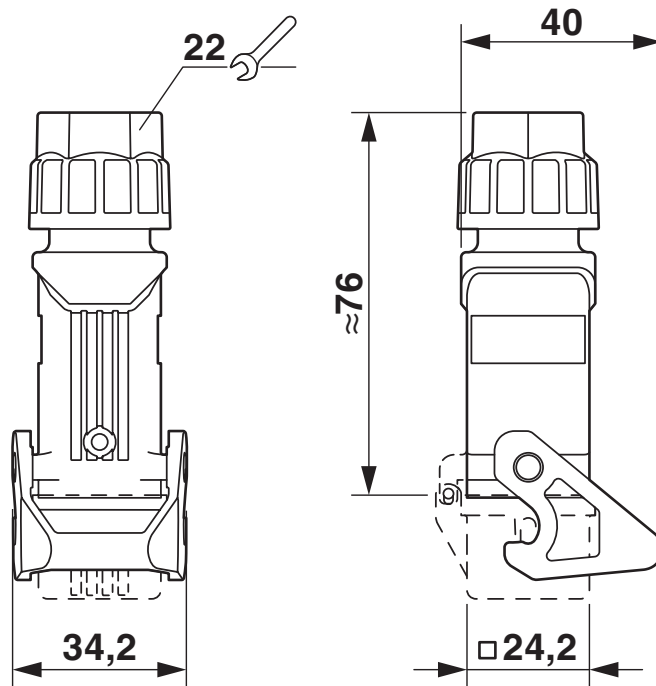
Maßzeichnung
