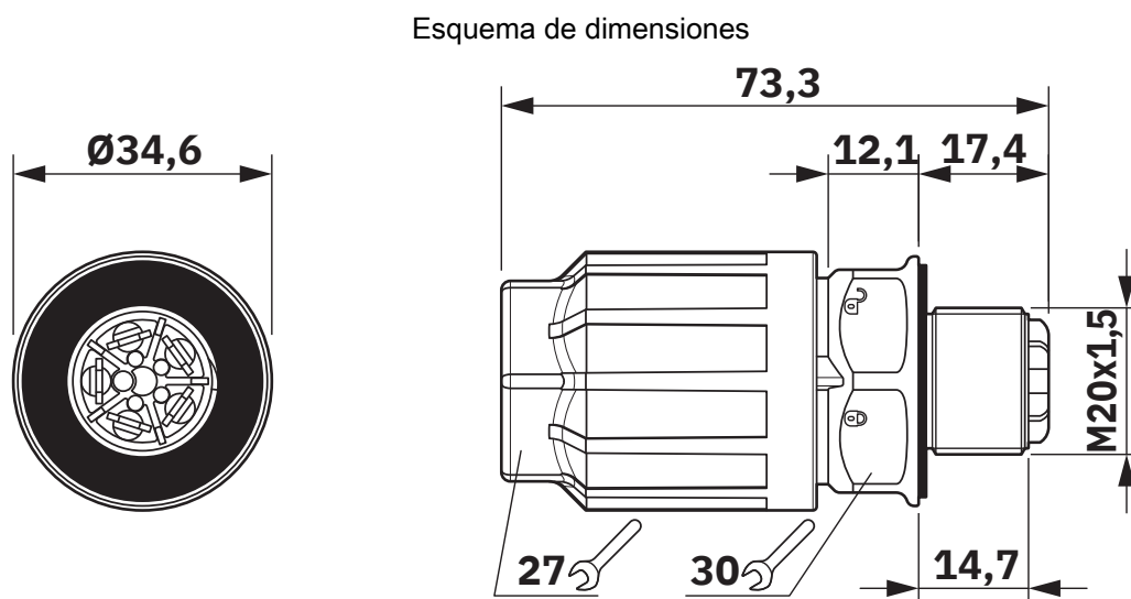
Dibujo acotado de QPD W 5 x 2,5 M20
