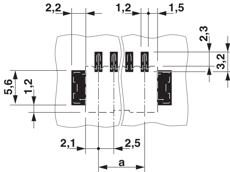
Bohrplan/Lötpadgeometrie
