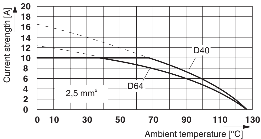
Courbe de derating pour 2,5 mm²
