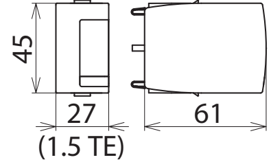
Maßbild DG MOD E CI WE 440
