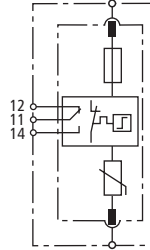
Prinzipialschaltbild DG MOD E CI WE 440
