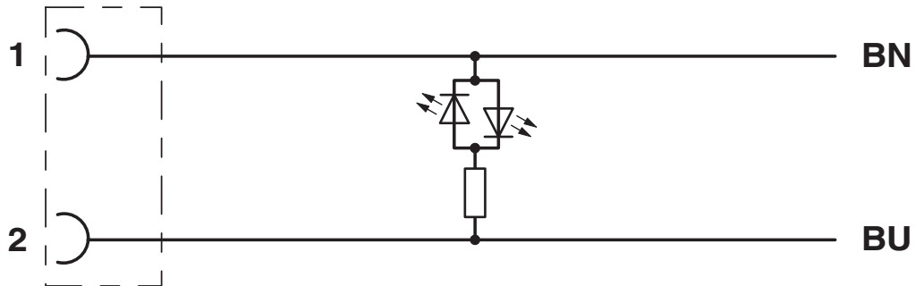
Diagrama eléctrico
