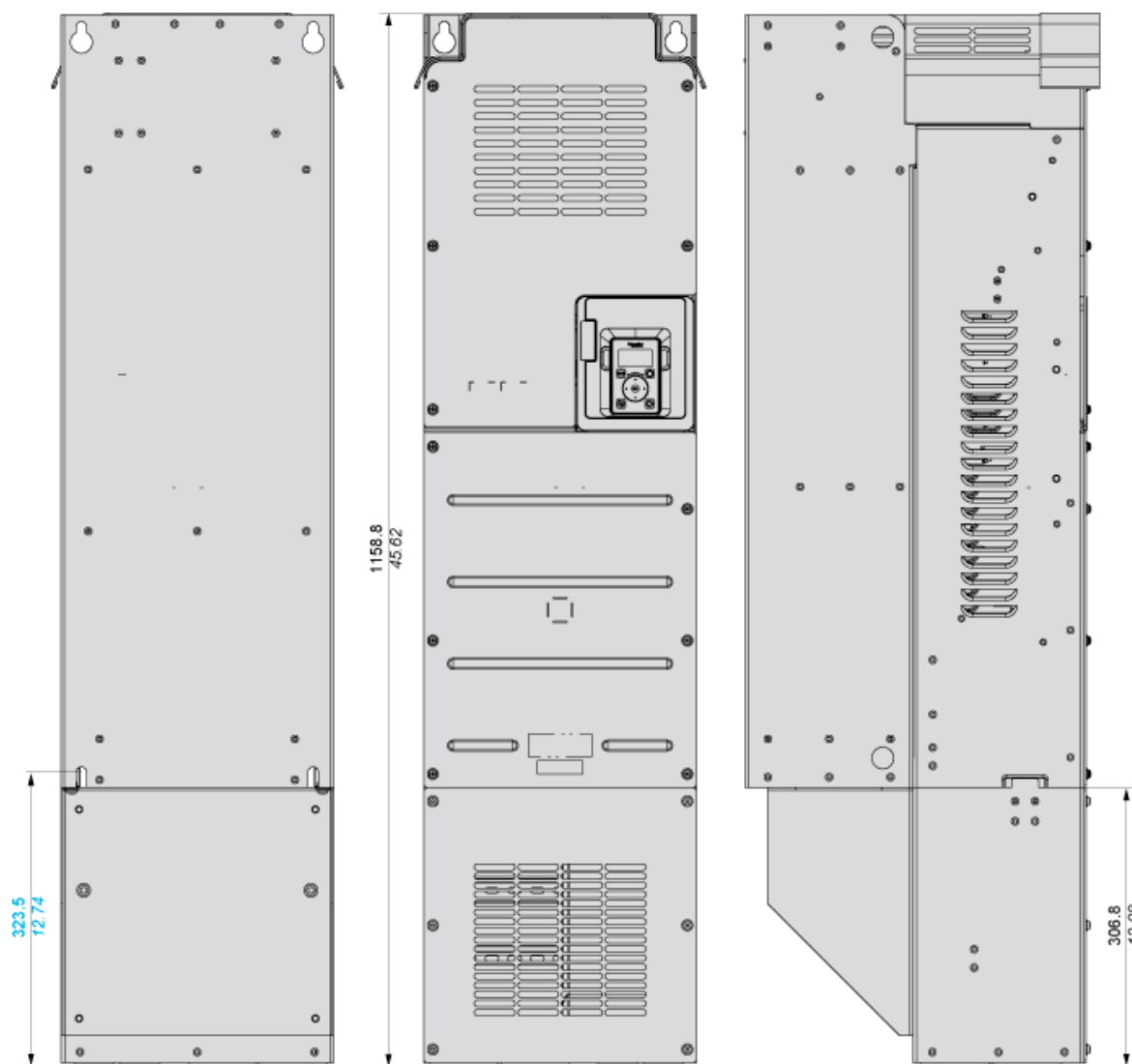
Disegni da sinistra a destra: vista posteriore, vista frontale e vista lato sinistro con coperchio superiore.
