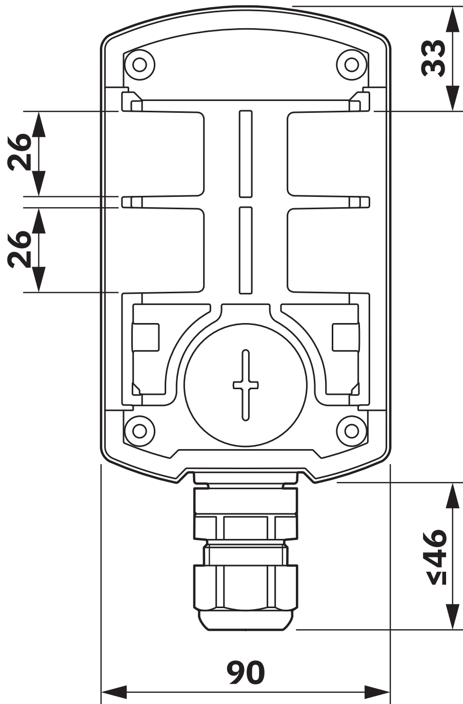
Maßzeichnung
