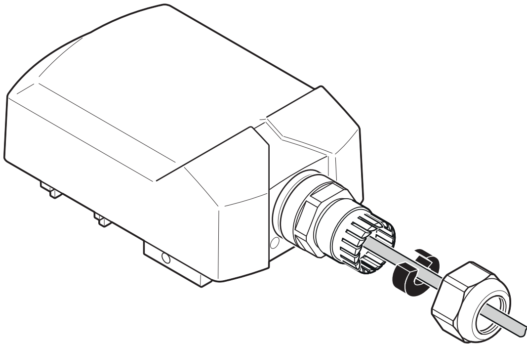
Schemazeichnung
