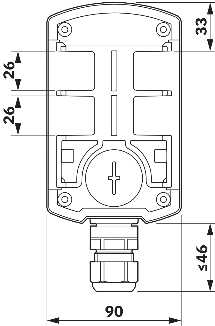
Dessin coté
