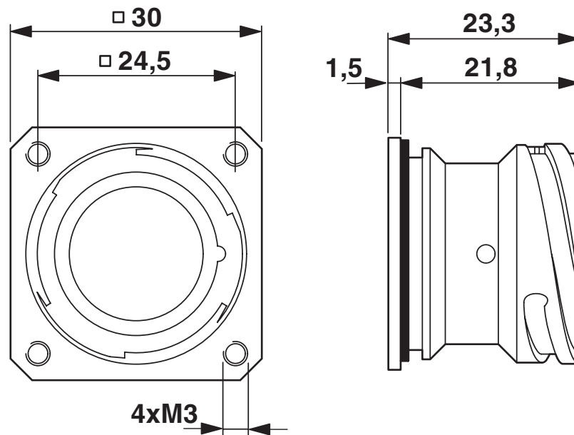
Maßzeichnung
