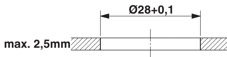
Maßzeichnung
