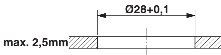
Dessin coté
