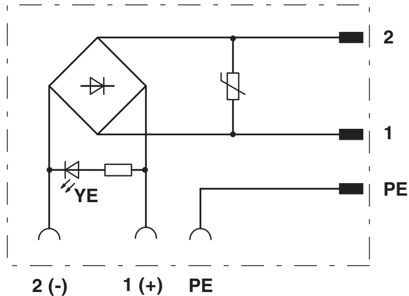
Diagrama eléctrico
