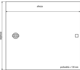
Dimensioni DPG LSA 60 P
