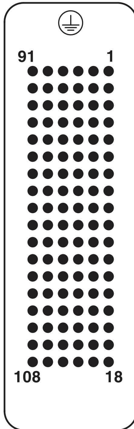
Schemazeichnung
