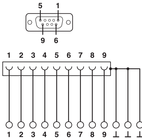
Diagrama eléctrico
