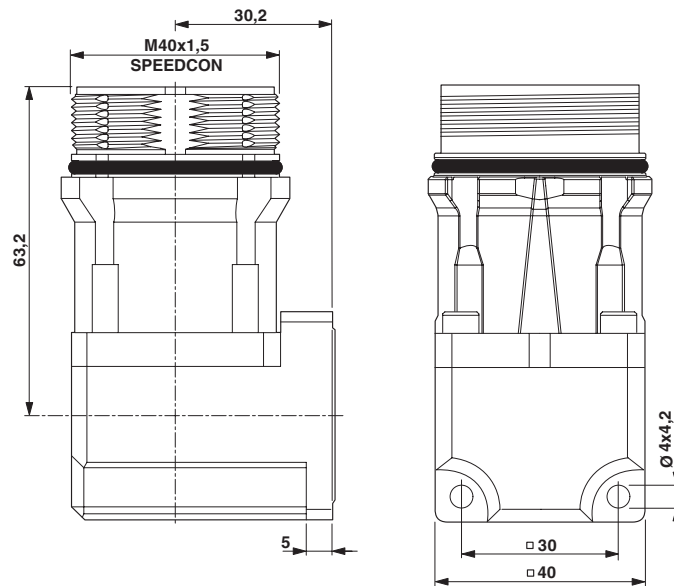
Maßzeichnung
