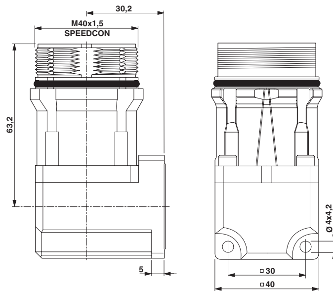
Dessin coté
