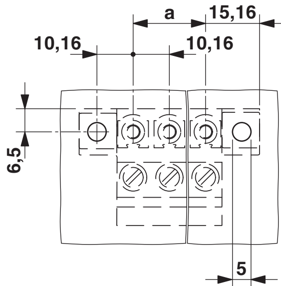
Bohrplan/Lötpadgeometrie
