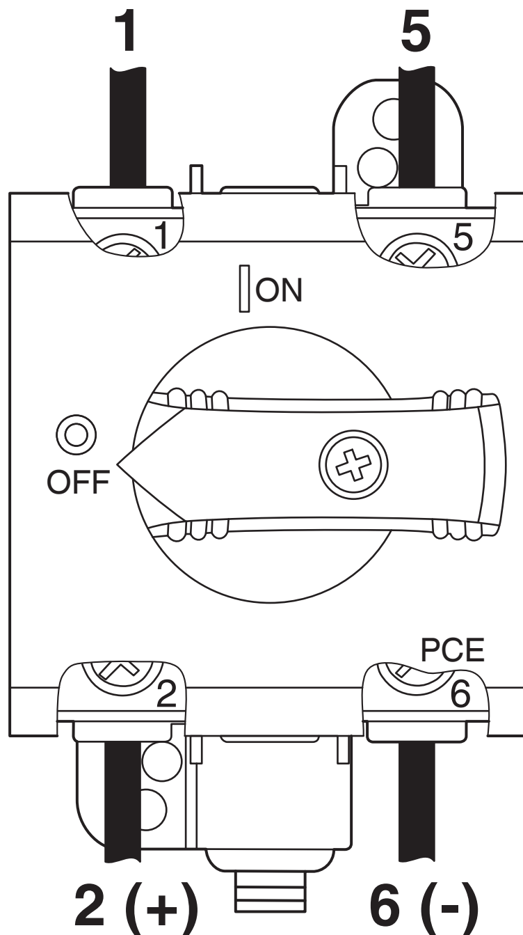
Anschlusszeichnung
