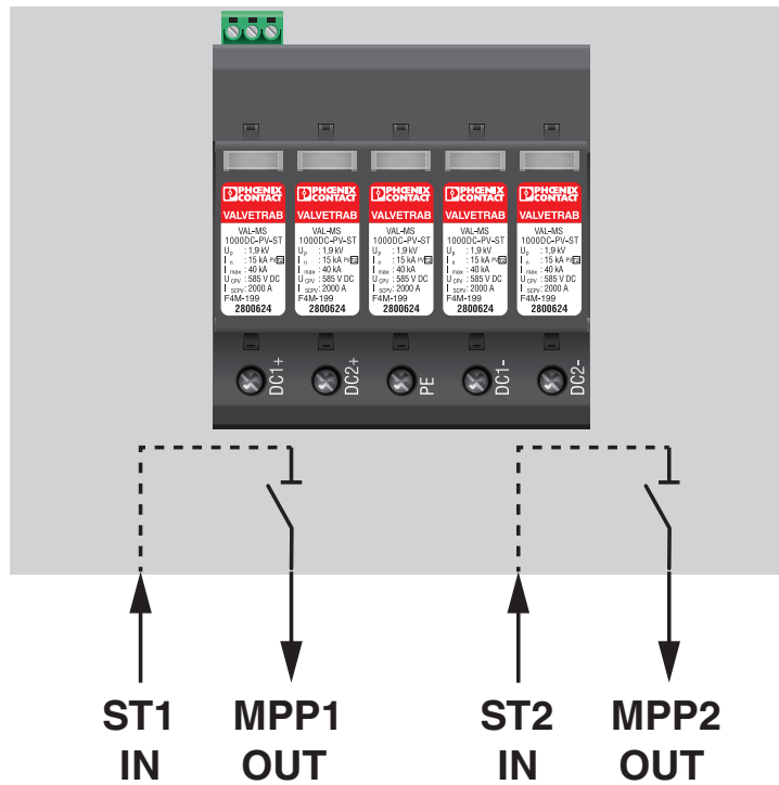
Anschlusszeichnung
