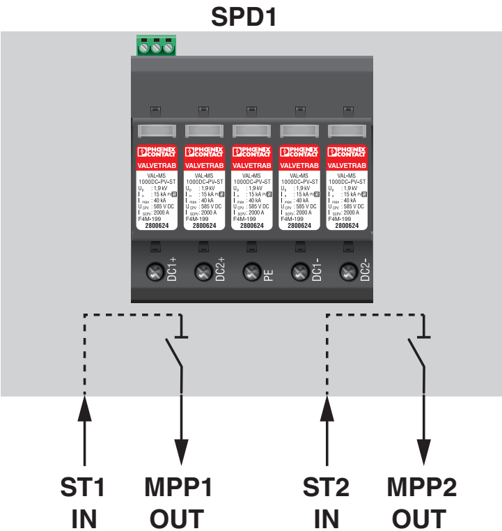
Dessin de la connexion
