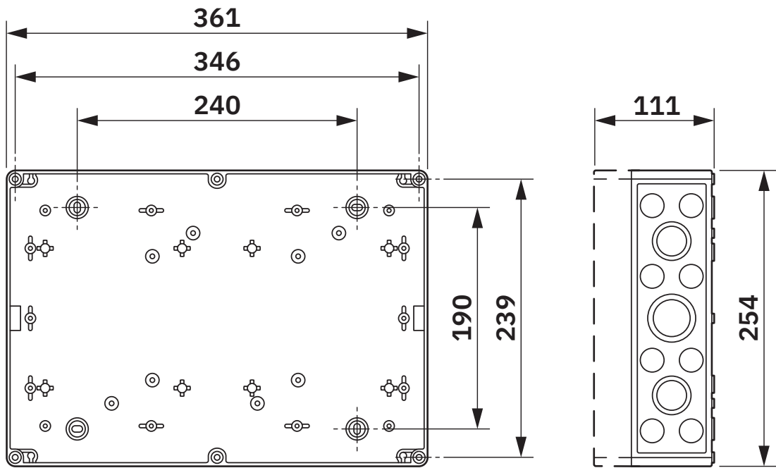
Dimensions du boîtier
