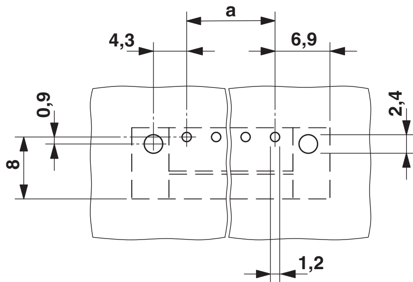
Bohrplan/Lötpadgeometrie
