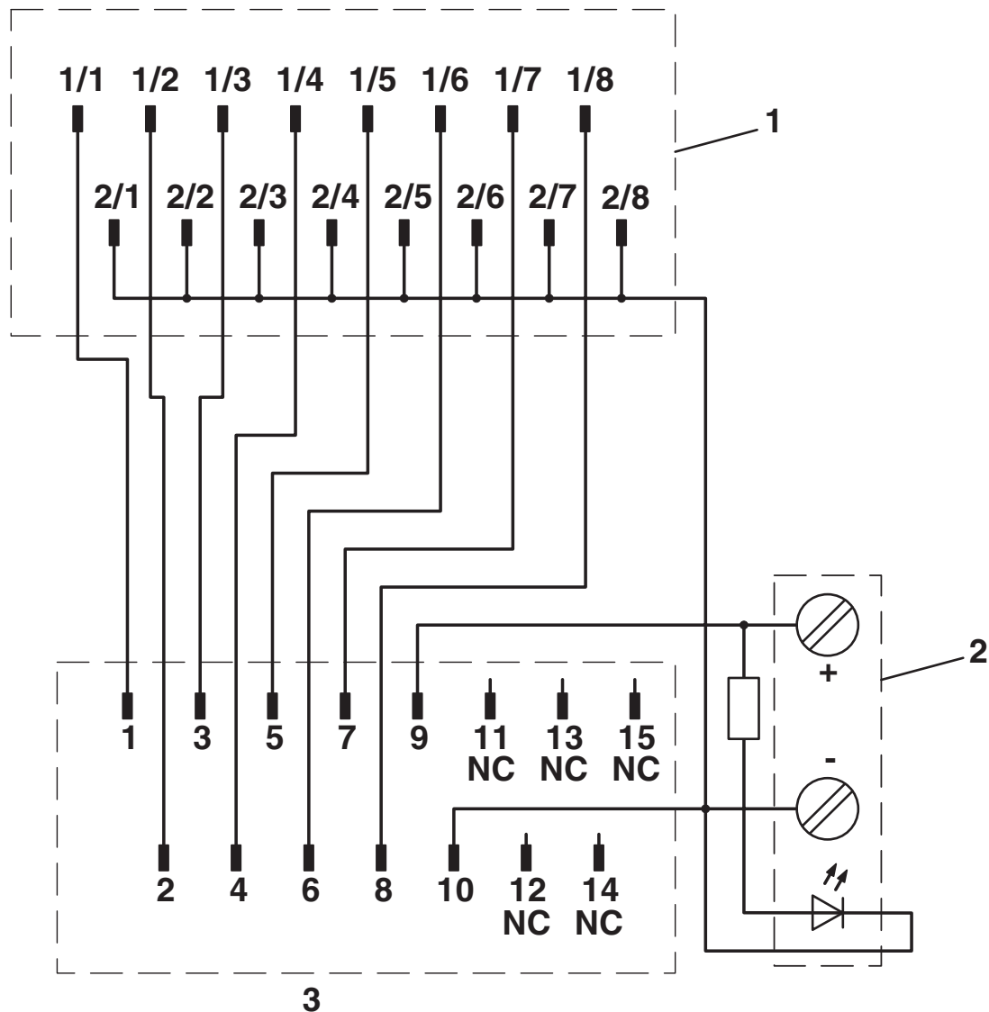
Diagrama eléctrico
