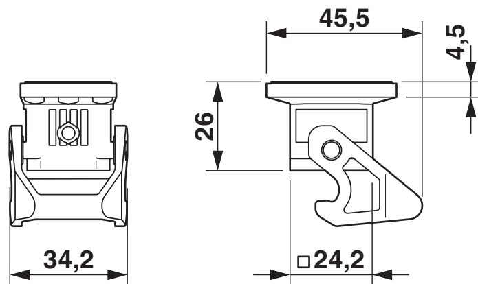
Maßzeichnung
