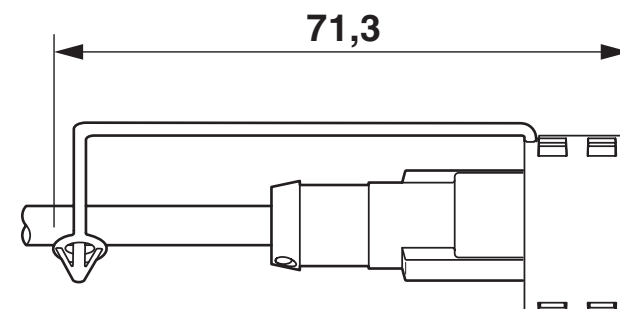
Dessin coté
