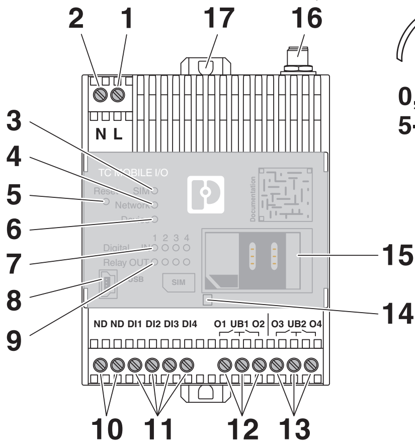
Dessin schématique
