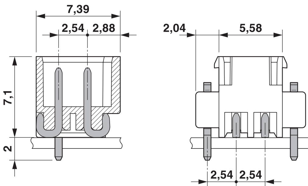
Dessin coté
