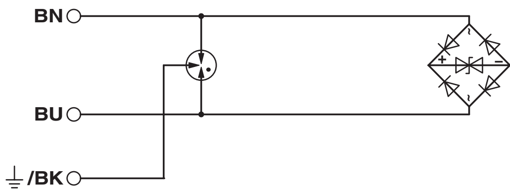
Schaltplan
