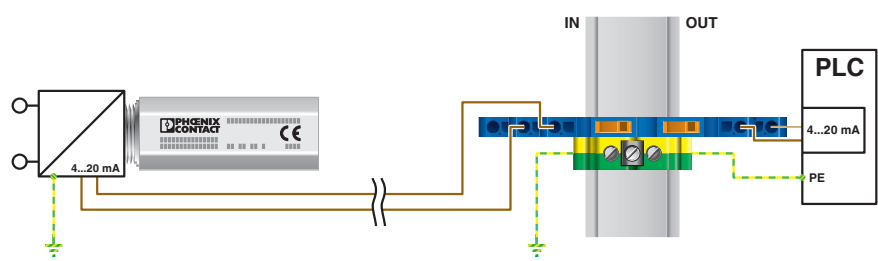
Applikationszeichnung
