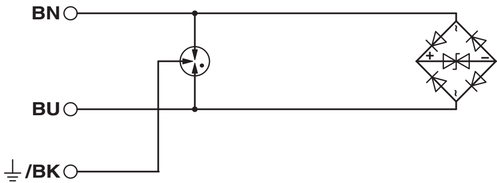
Diagrama eléctrico
