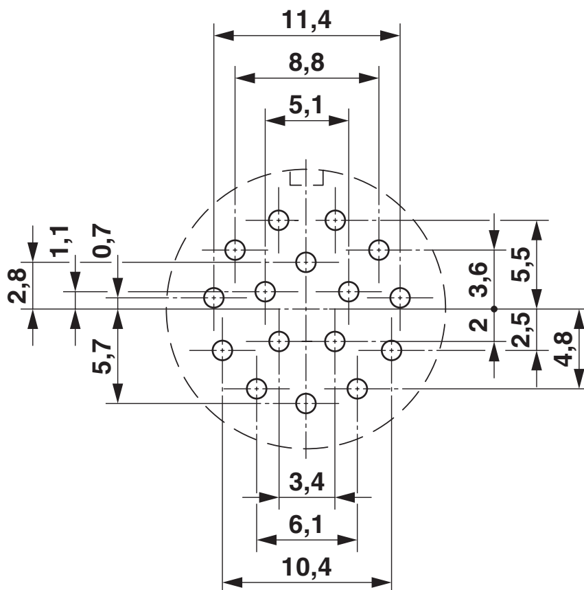
Bohrplan/Lötpadgeometrie
