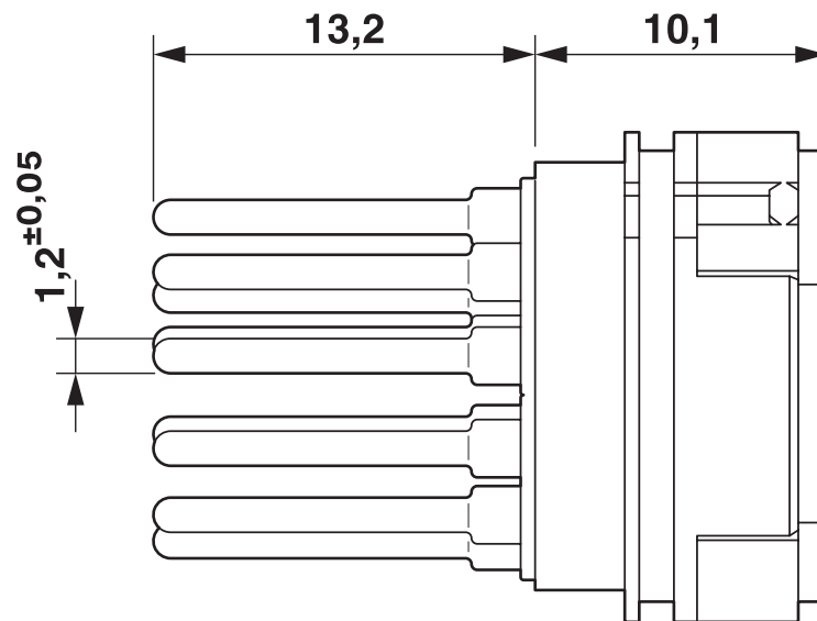
Maßzeichnung
