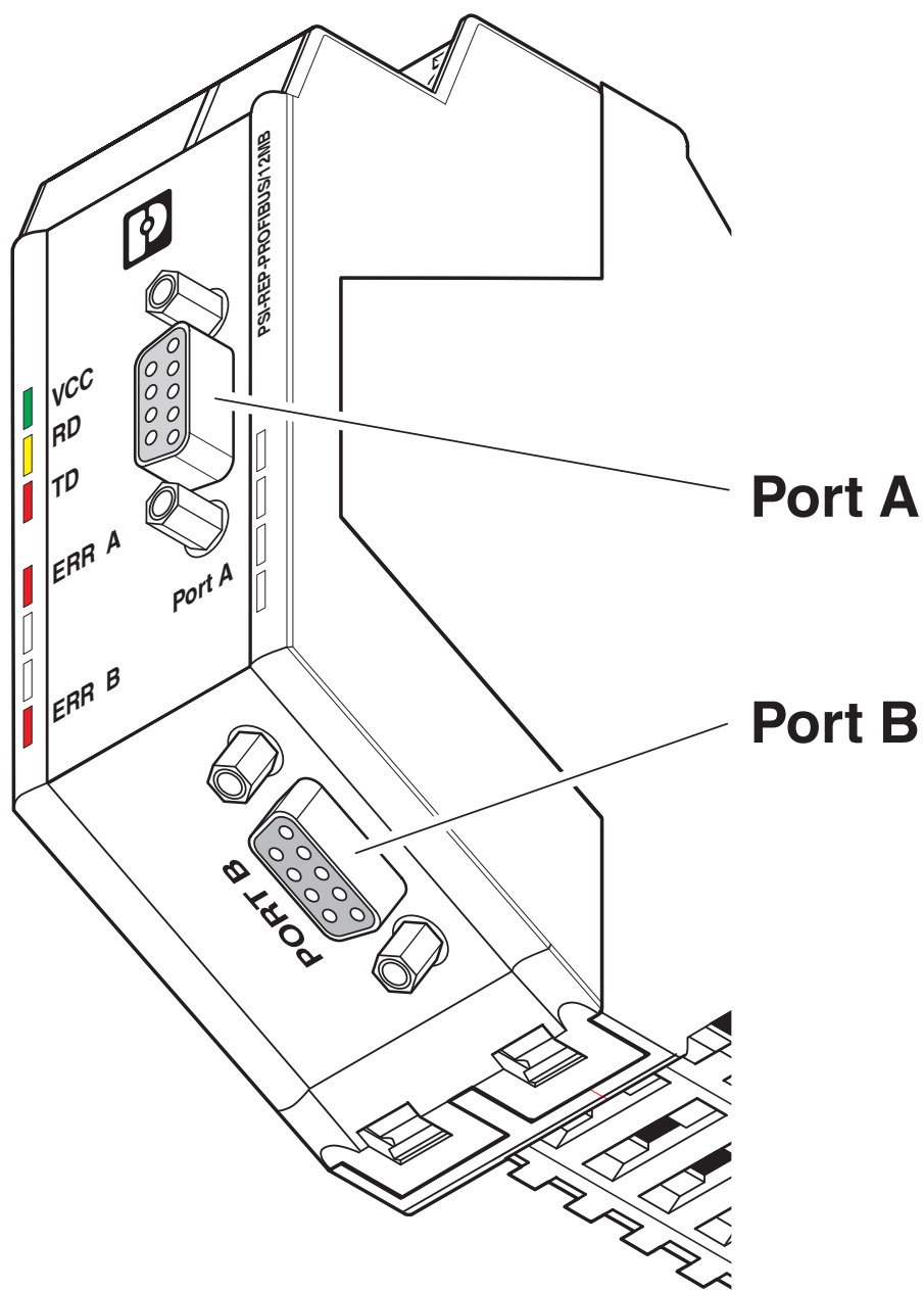
Plano esquemático
