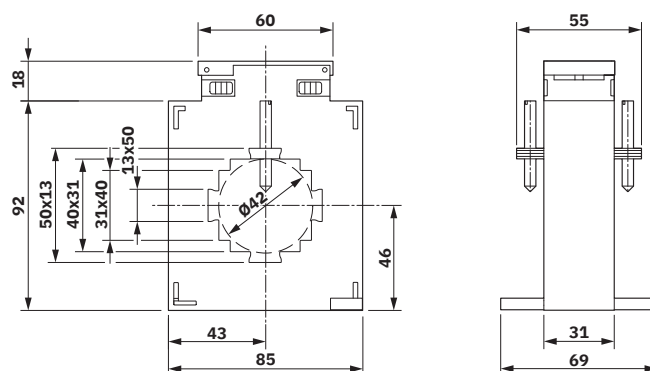
Dessin coté
