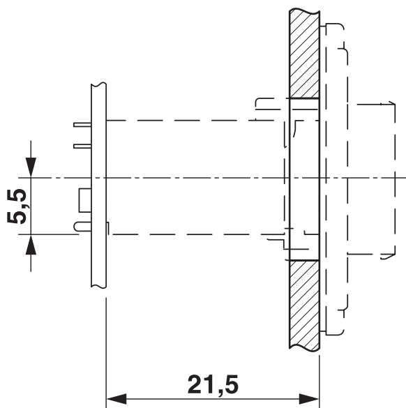
Dessin coté
