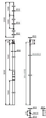
Maßbild HVI 23 L6M SR3200 IP RFS2500
