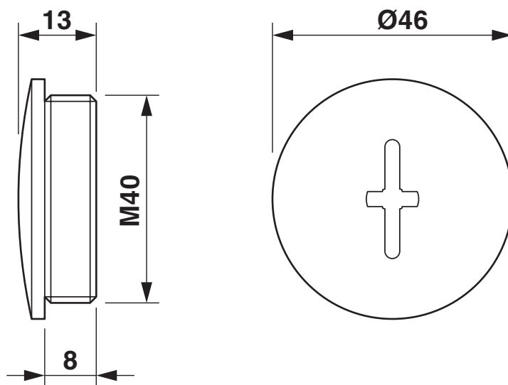
Esquema de dimensiones
