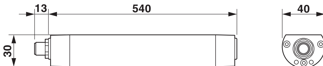
Dessin coté
