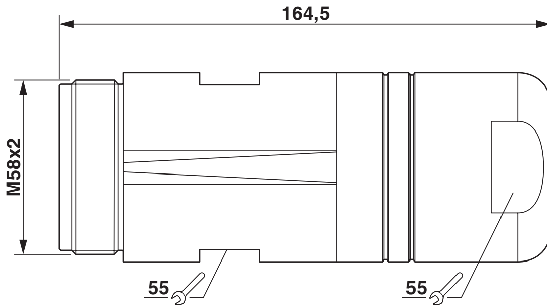
Maßzeichnung
