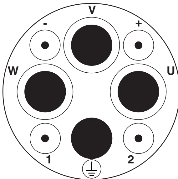
Schemazeichnung
